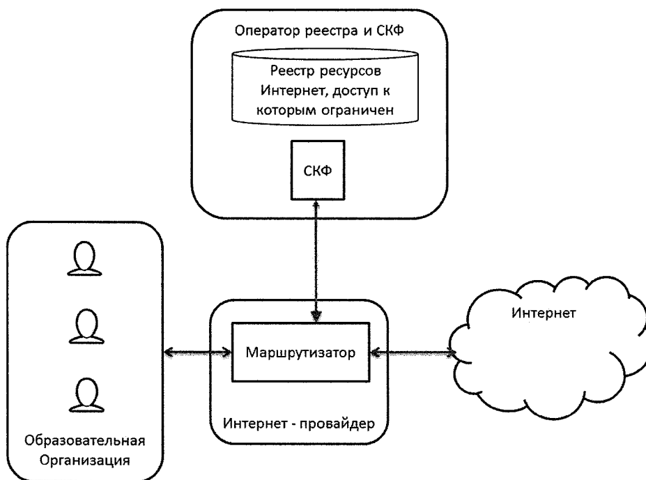
Рисунок 5. Схема работы контент-фильтрации при едином решении
